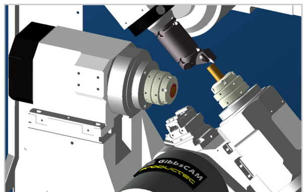
Dockning av detalj från huvudspindel till subspindel och svarvning med tiltad B axel samt tiltad subspindel.
