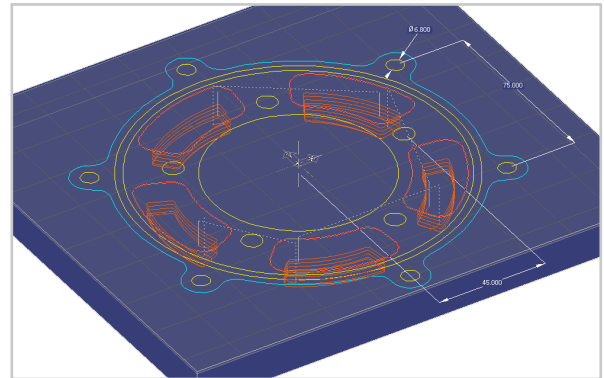
2D ritning samt rektangulärt råämne skapat i GibbsCAM. Mått och håldimensioner ändras enkelt med hjälp av GibbsCAM's "Geometry Expert" Ovan: valsfräsning av sex fickor, med spiralnedmatning.
