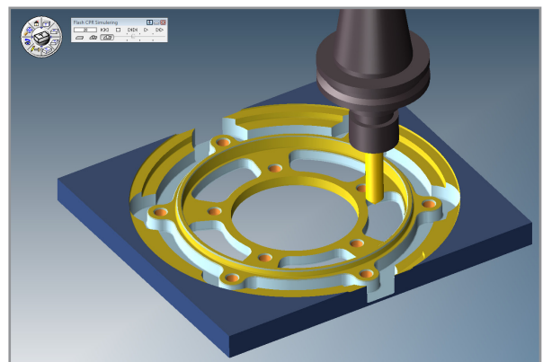
Bearbetningen verifieras i den inbyggda 3D simulatorn. Verktygsbanorna omvandlas slutligen till optimerad NC-kod för valfritt styrsystem, med borrar-cykler & underprogram för enklare hantering i maskin.
